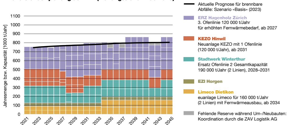
Abb. 5.1 Mengenzenario Basis in der aktualisierten Kapazitäts- und Standortplanung der KVA (Planungsstand Ende 2023)
