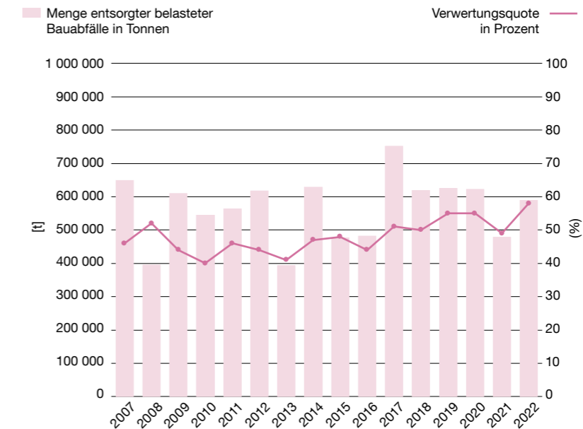
Abb. 6.1 Mengen und Verwertungsquote verschmutzter Bauabfälle von belasteten Standorten
