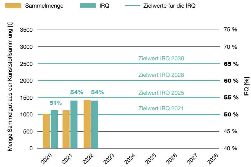
Abb. 4.1 Menge gesammelter Kunststoffabfälle aus Haushalten und industrielle Rückführungsquote (IRQ)
