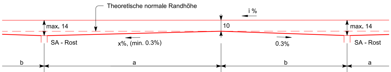
Maximale Strassenablauf - Abstände (bei Randgefälle 0.3%)
